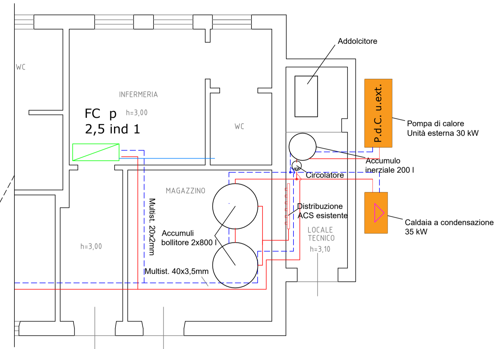
INGRANDIMENTO Scala 1:50
