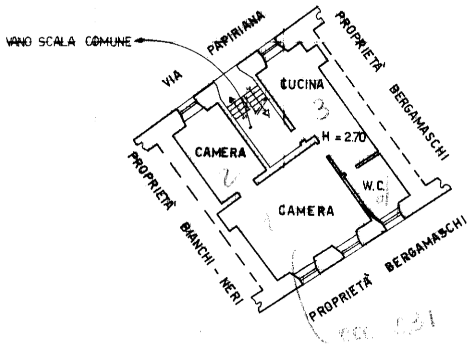
PIANTA PIANO TERRENO
